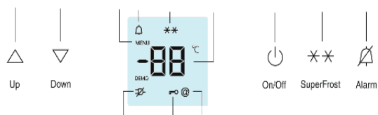
Schema del display (tranne 2477)
